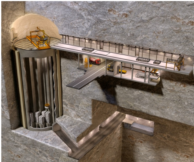
Figur 5-3. Siloförvaret i befintligt SFR under driftskedet.
