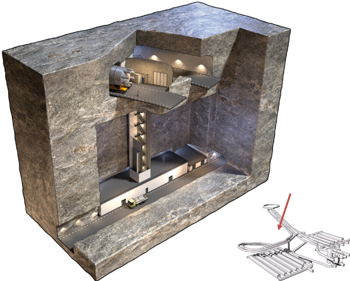
Figur 5-5 Teknikinstallationstunnel, TIT, i utbyggd del av SFR.
