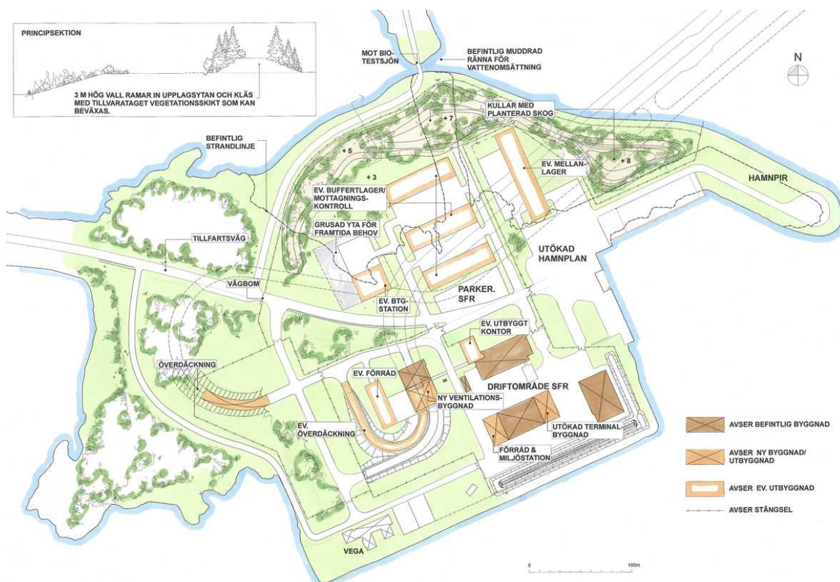
Figur 5-1 Principskiss över SFR:s ovanjordsdel.
