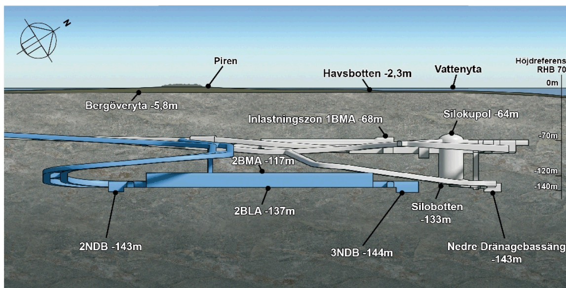
Figur 5-4 Höjdrelationer, blå färg avser utbyggd del.
