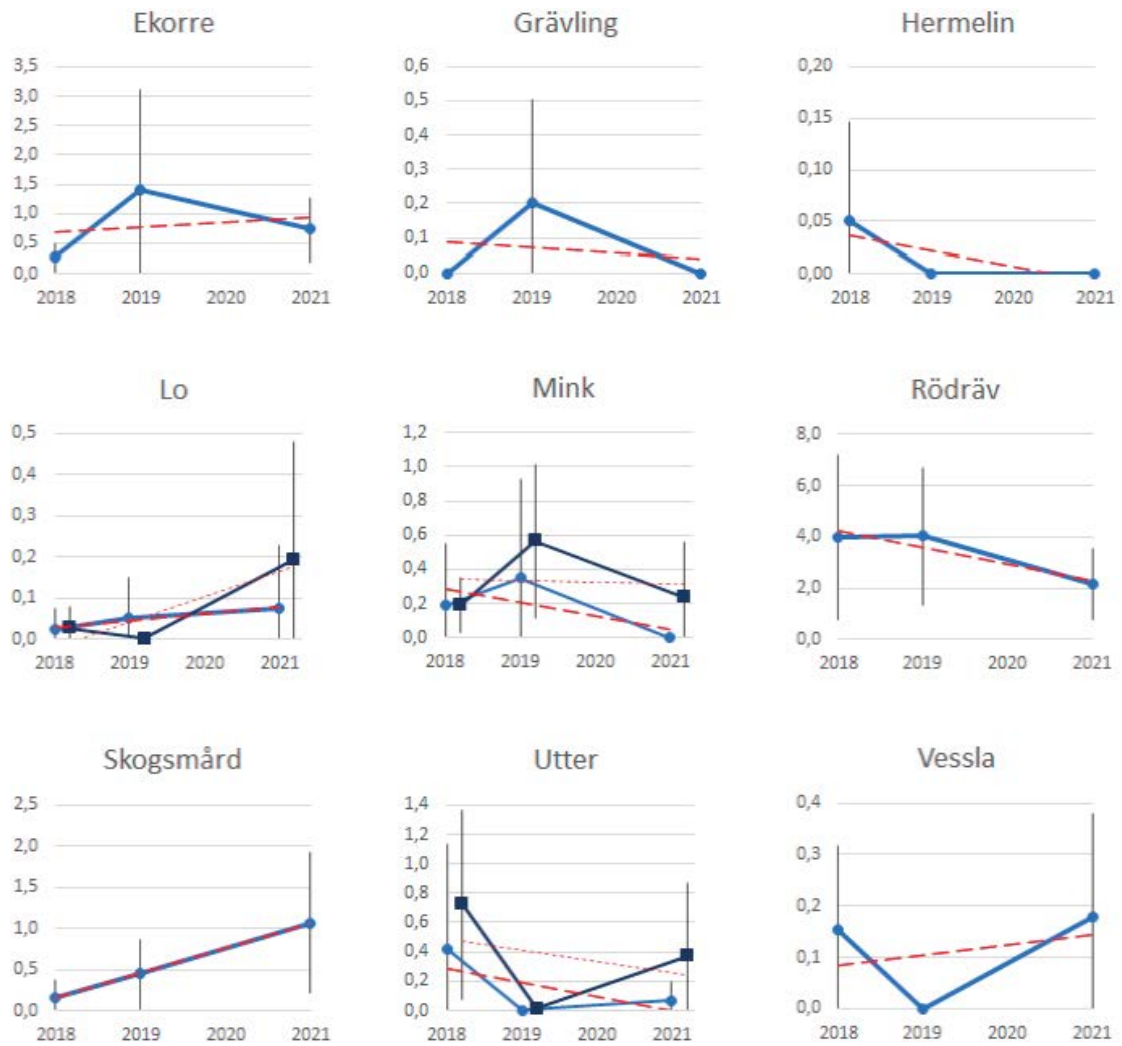
Figur 3-7. Populationsutveckling hos ett antal rovdäggdjur i Forsmark utifrån spårinventering längs räta linjer på fastmark (ljusblå linjer) och längs vattenlinjer (mörkblå linjer). Arter där ingen positiv observation gjorts har utelämnats – brunbjörn, bäver, iller och varg. Inte heller hund och katt redovisas grafiskt. Svarta vertikala staplar genom punkterna indikerar 95 % konfidensintervall. Streckade röda linjer indikerar linjära trender.
