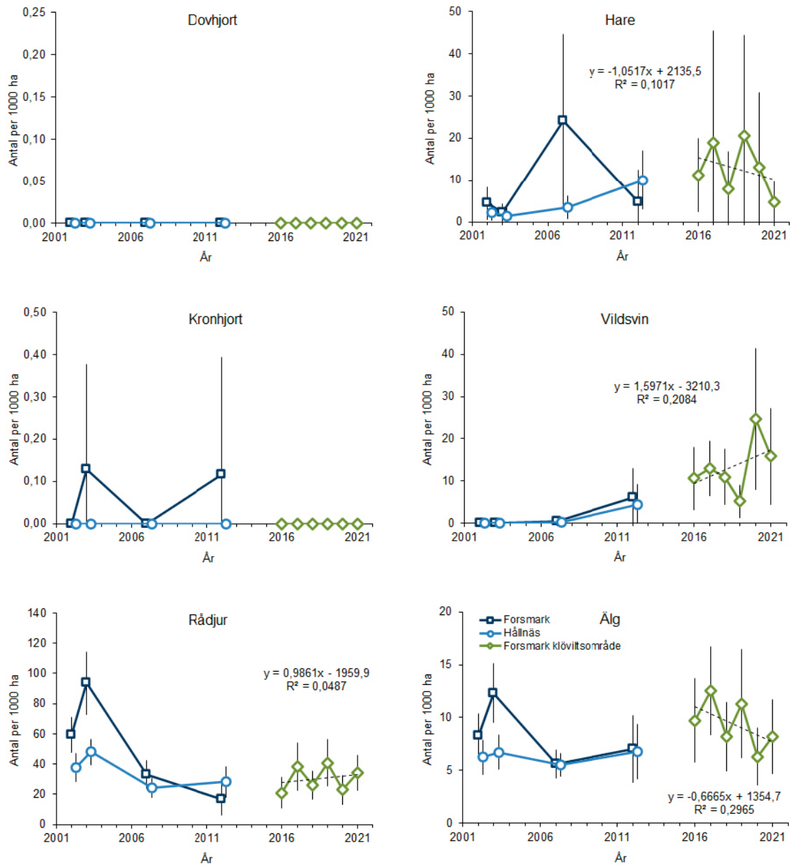
Figur 3-2. Populationsutveckling hos dovhjort, hare (fälthare och skogshare), kronhjort rådjur, vildsvin och älg baserat på spillningsinventering 2002–2012 i Hållnäs (ljusblå linje) och Forsmark (mörkblå linje) och från 2016 och framåt i Forsmarks klöviltssområde (grön linje). Svarta vertikala staplar genom punkterna indikerar 95 % konfidensintervall.
