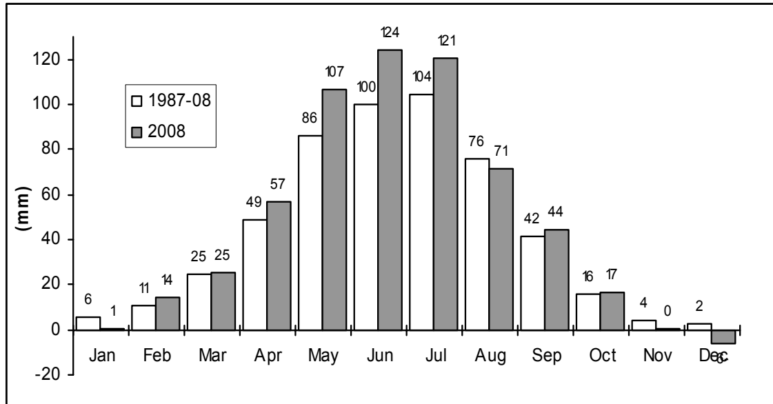
Figure 5-6. Potential evapotranspiration. Monthly values for Norra Äspö 2008 and monthly means from Norra Äspö, Gladhammar and Ölands Norra Udde 1987 – 2008.
