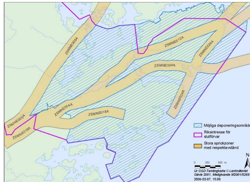
Figur 3-4. Tillgängliga ytor för deponeringsområden.
