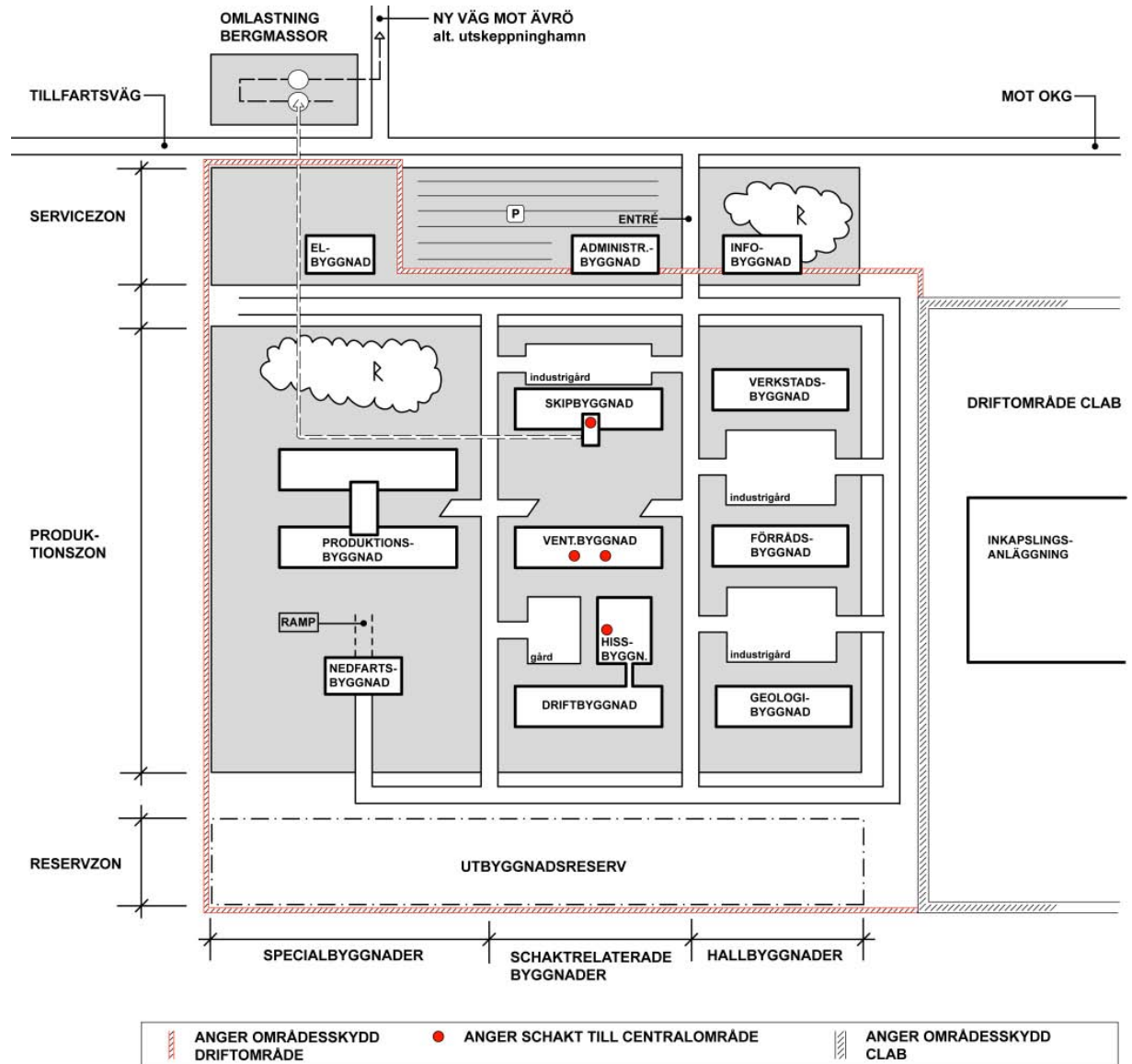
Figur 4-2. Dispositionsplan för driftområde – Läge Clab.
