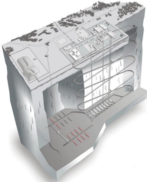
Figur C-3. Inledande drift.
