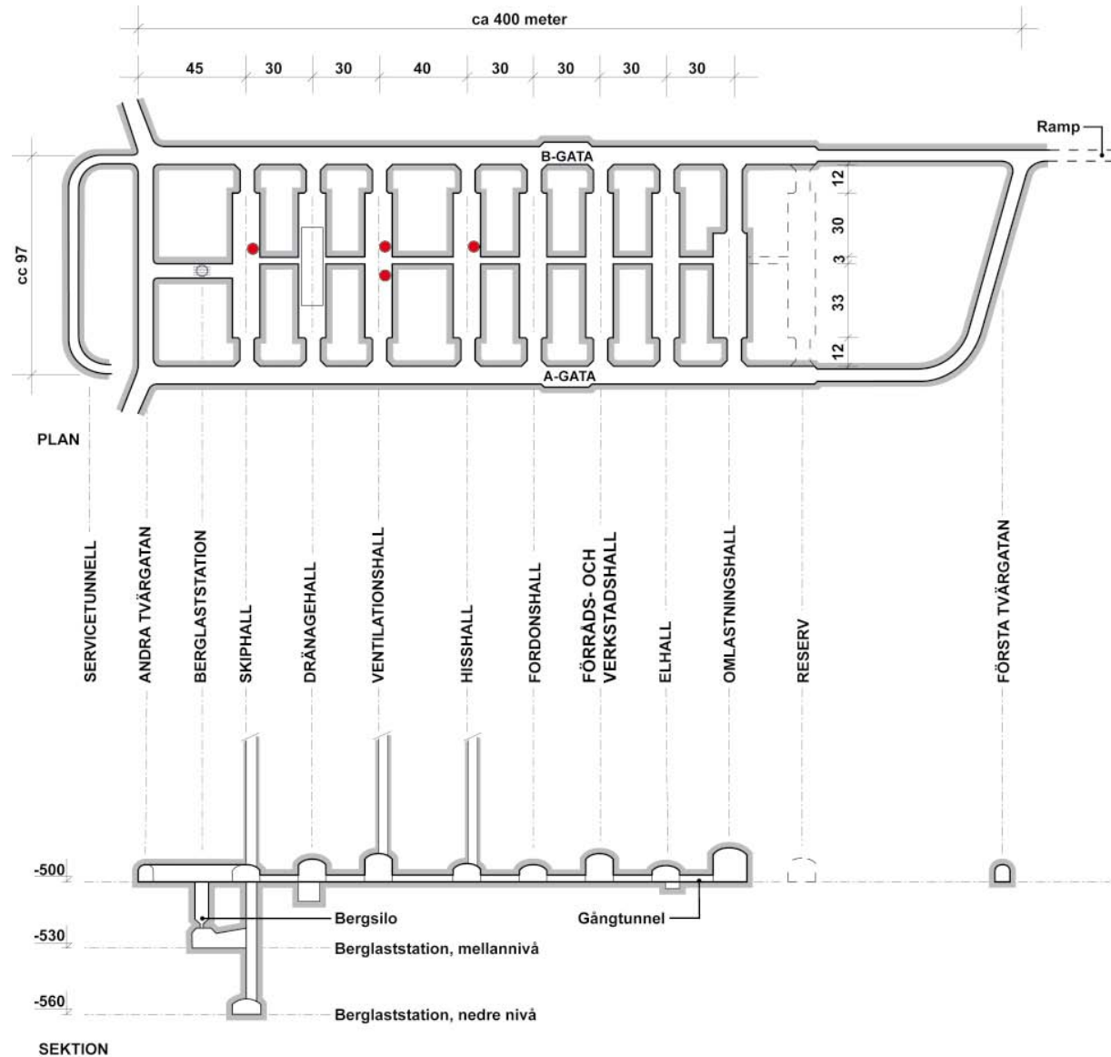
Figur 4-5. Dispositionsplan för centralområde – Läge Clab.
