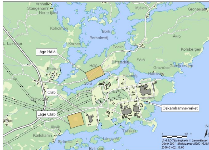
Figur 3-7. Läge Clab och Hålö.
