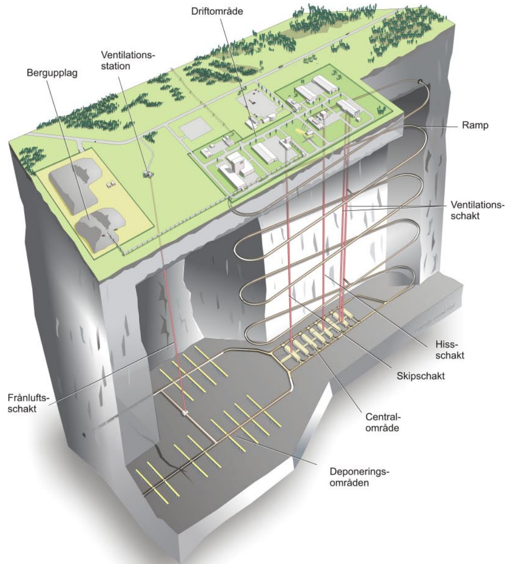
Figur 1-2. Slutförvarsanläggningen.
