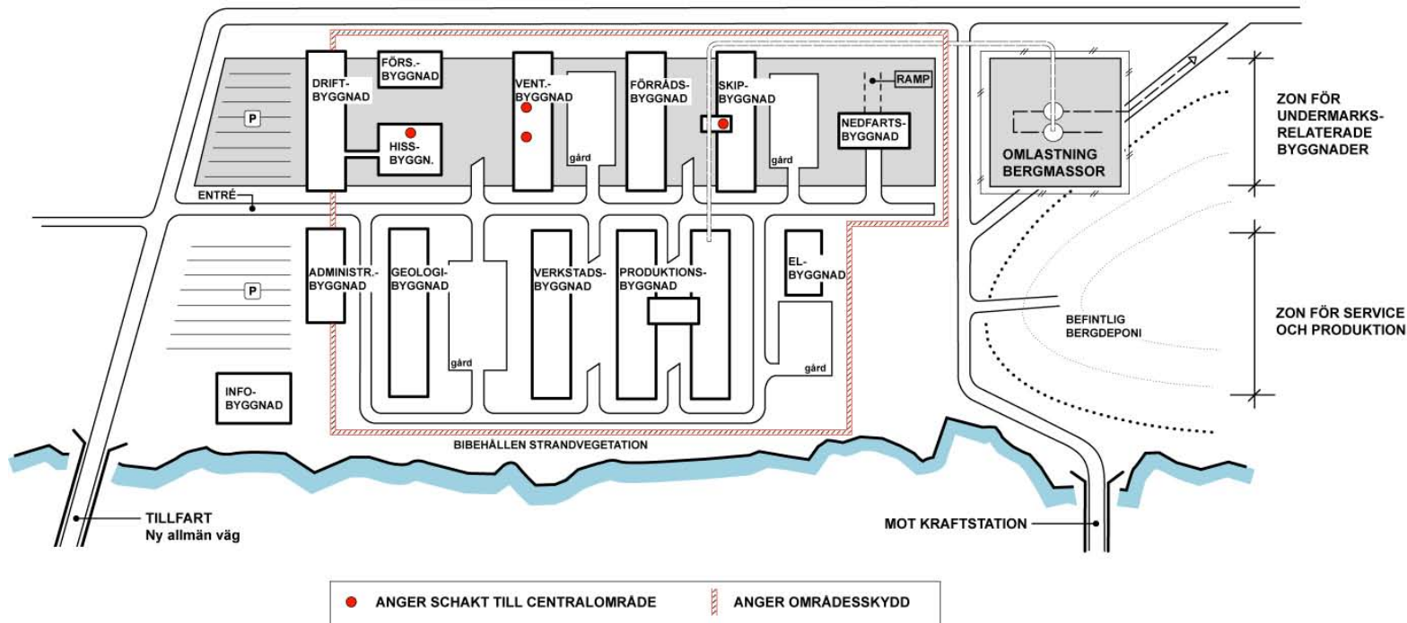
Figur 5-2. Dispositionsplan för driftområde – Läge Hålö.
