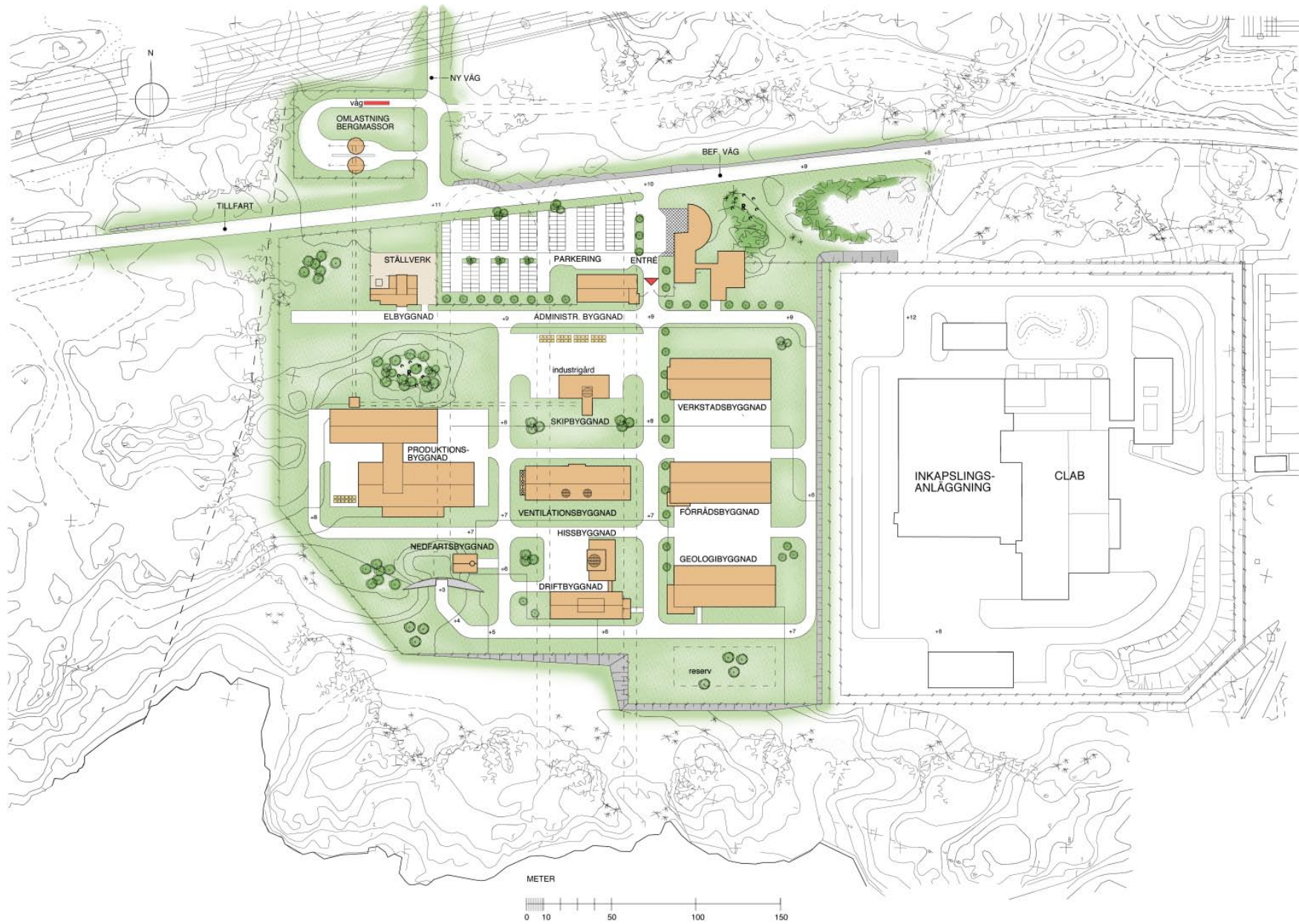
Figur 4-4. Situationsplan för driftområde – Läge Clab.
