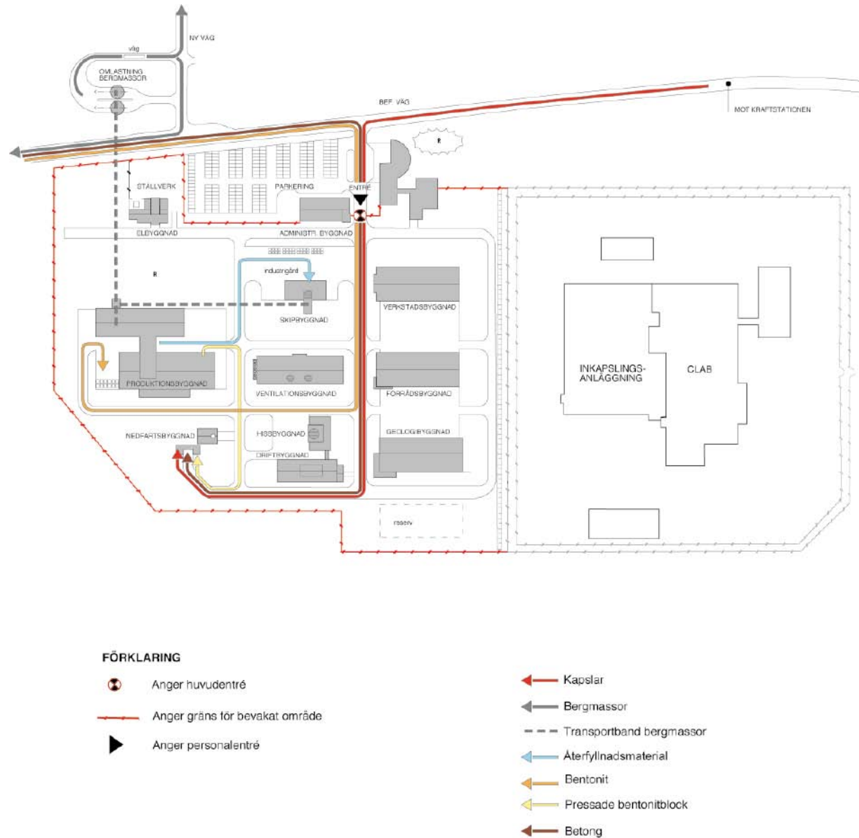
Figur 4-3. Fysiskt skydd och interna transporter – Läge Clab.
