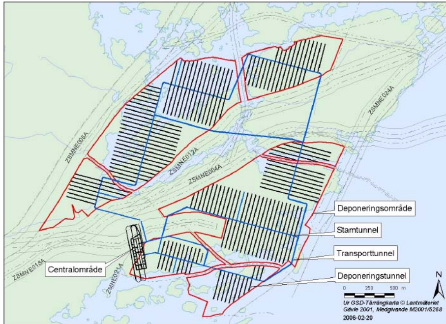
Figur 4-6. Undermarkslayout – Läge Clab.
