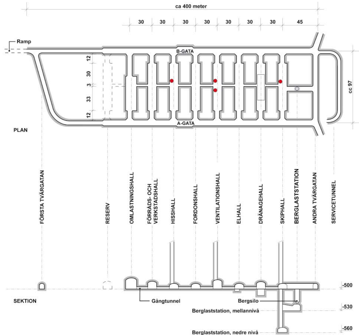
Figur 5-5. Dispositionsplan för centralområde – Läge Hälö.
