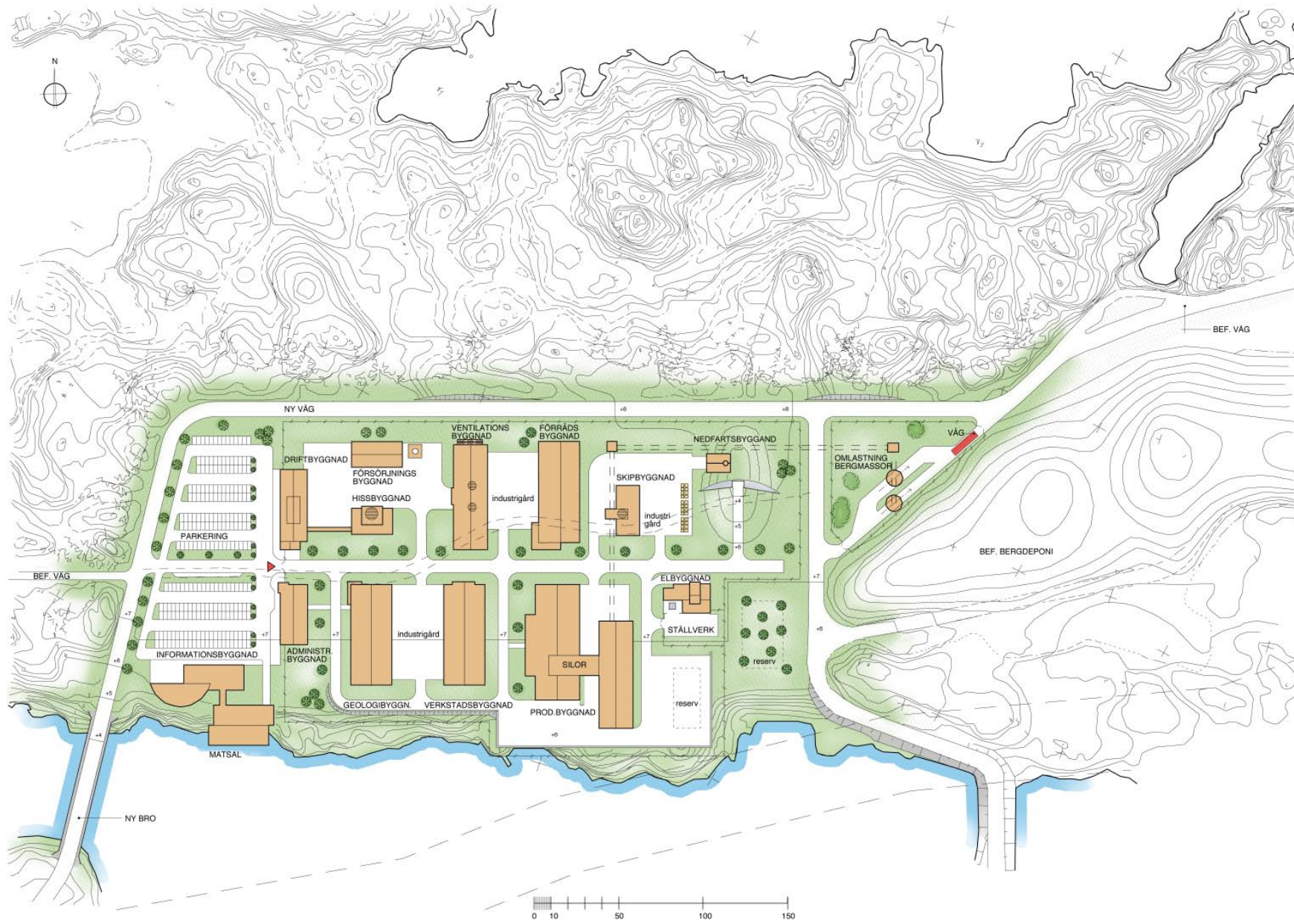
Figur 5-4. Situationsplan för driftområde – Läge Hälö.
