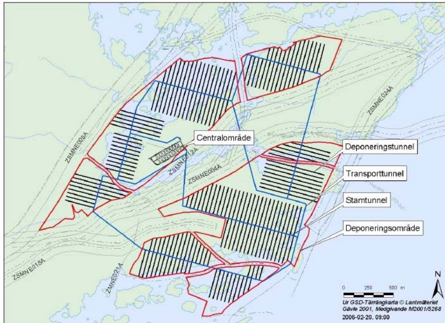
Figur 5-6. Undermarkslayout – Läge Hälö.
